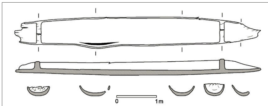
Toušeňský monoxyl (dle ROGERS Jason Samuel, Czech logboats. Early inland watercraft from Bohemia and Moravia . In: Sborník prací filozofické fakulty brněnské univerzity , 2011, roč. 16, s. 185)
